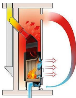
TOPLOZRAČNI KAMIN
